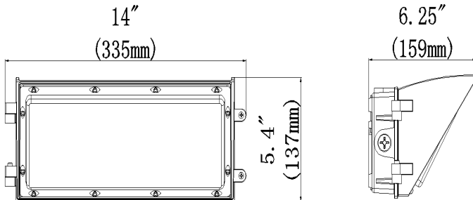
GWL-HWP-45-PF-XX-C
